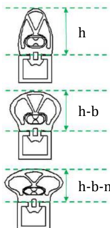
Abbildung 2: Skizze Schaltleiste
