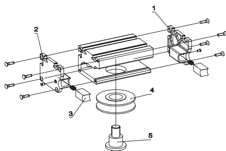
Zentrischer Bolzen
