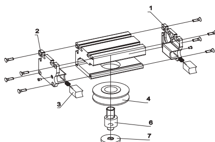
Boulon excentrique
